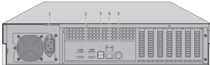
图1-3 TL-TUMS2700后面板示意图
